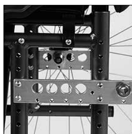
MG 86 Drivhjulsinfästning aktiv/passiv
