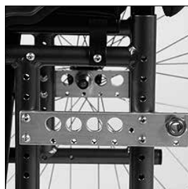
MG 86 Drivhjulinfästning aktiv/passiv
